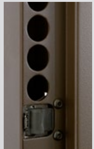
Sistema antitarjeta y regulación del resbalón
