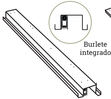
Carenado Inferior
