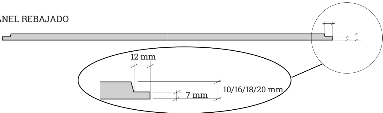
PANEL ESTÁNDAR
